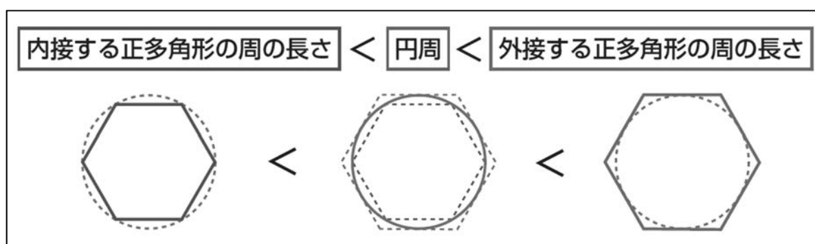
図1 円に内・外接する多角形の周の長さとの関係
