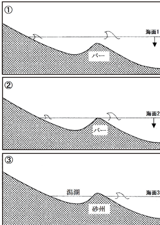
図3 海底砂州（バー）の離水によって砂州が形成されるとの説を示す模式図。海水準が低下すると（①→③）、バーが海面上に現れる。
