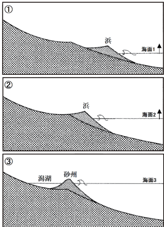
図4 海水準の上昇（①→③）に伴う浜の陸側・上方への移動と成長によって砂州が形成されるとの説を示す模式図。
